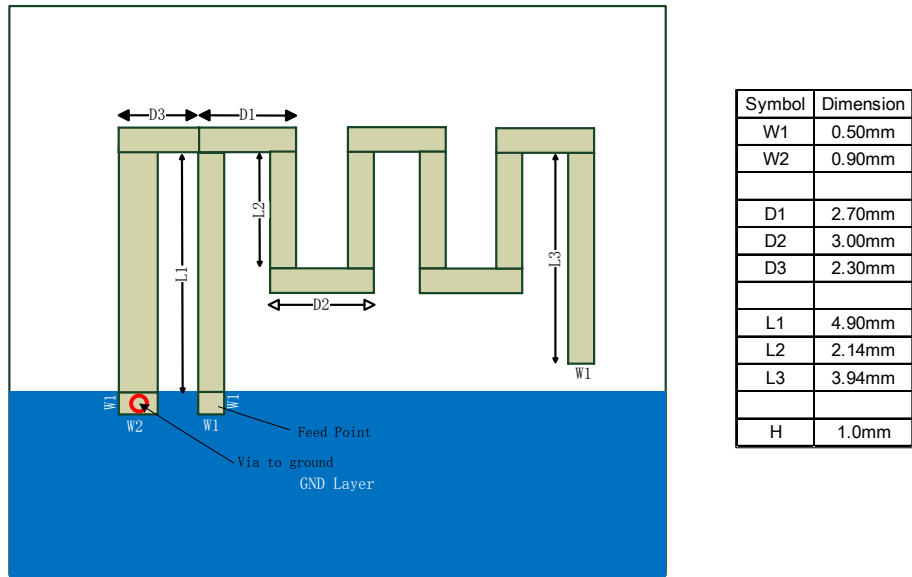
图 1-13 PIFAA 型天线结构尺寸图
