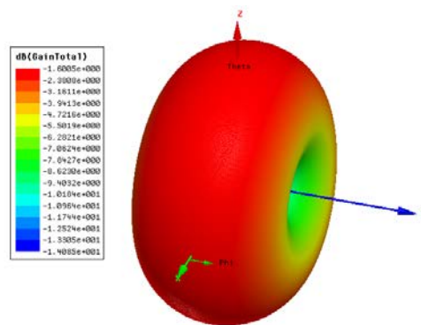
图 1-24 PIFA C 型天线 3D 增益图
