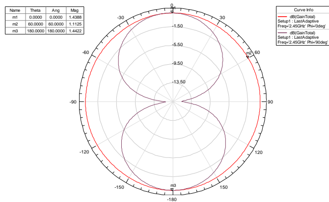
图 1-3 Wiggle A 型天线 2D 增益图
