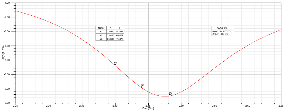
图 1-10 Wiggle C 型天线 S11 参数图
