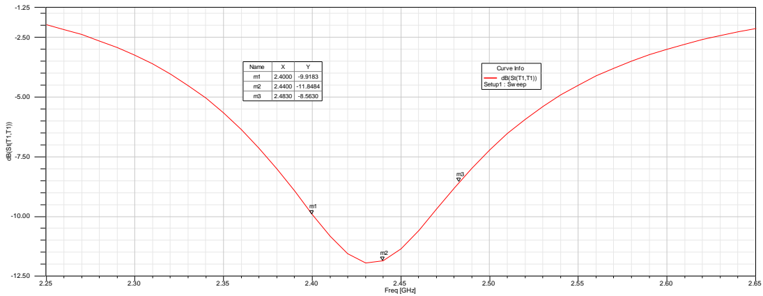
图 1-18 PIFA B 型天线 S11 参数图
