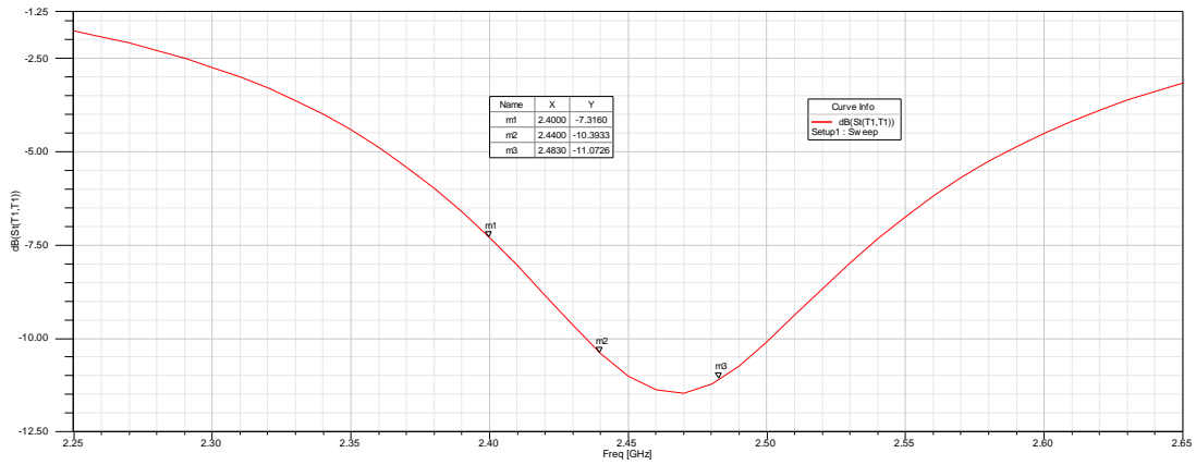
图 1-2 Wiggle A 型天线 S11 参数图
